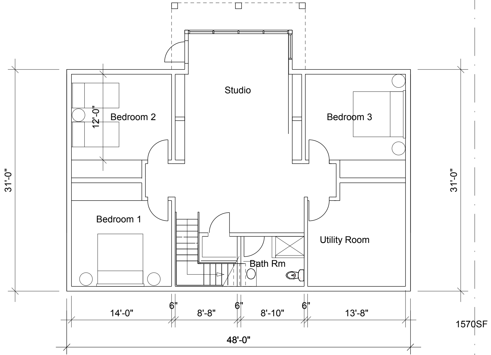
LOWER LEVEL PLAN SCALE: 1/8" = 1'-0"
